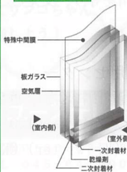
防犯ガラスの効果
