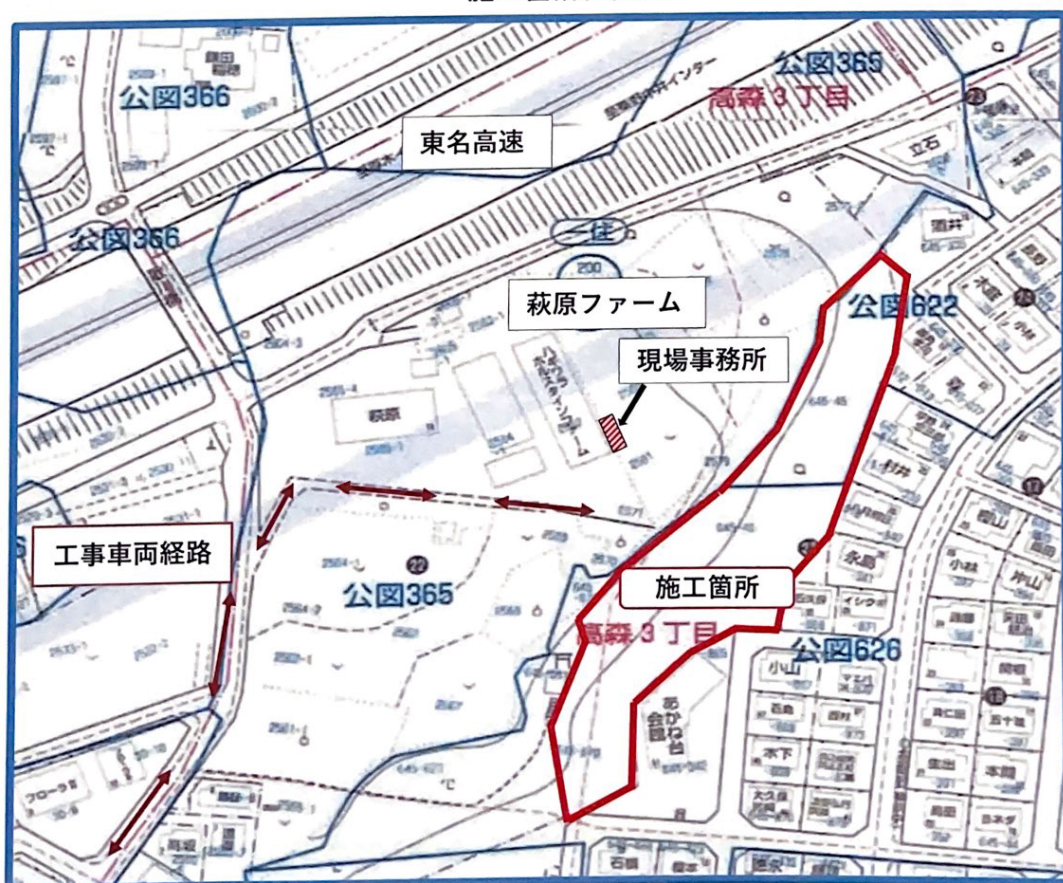
施工箇所位置図
